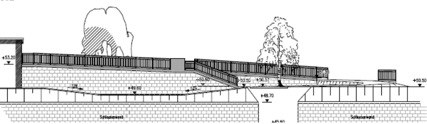
Ansicht Wasserkunst
