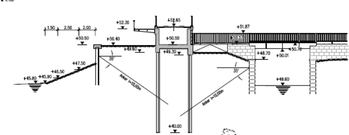
Schnitt 2-2
