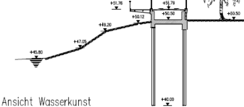
Ansicht Wasserkunst
