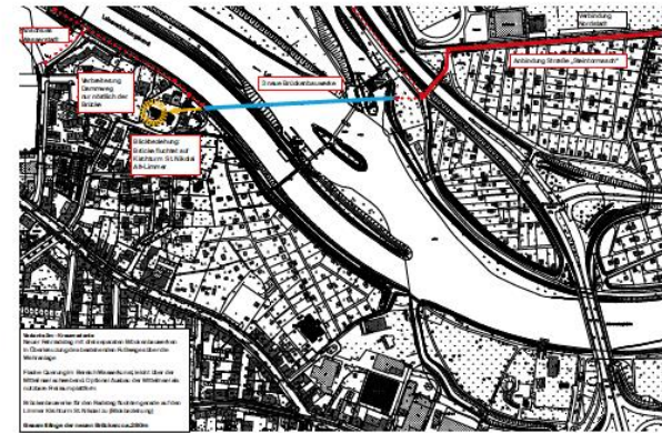
Fussgänger- und Radfahrerbrücke an der Wasserkunst - Variantenbetrachtung Variante 1a - Wehrquerung
