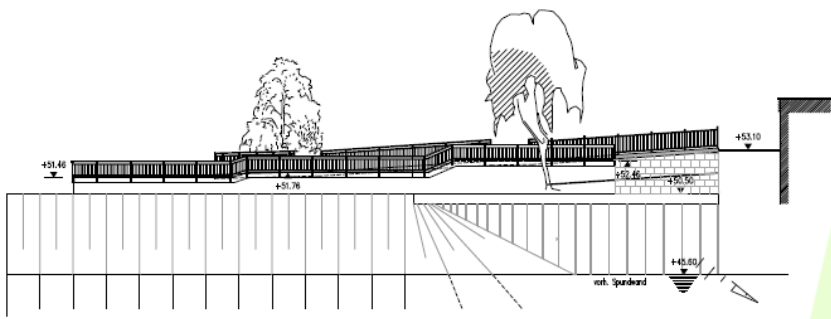
Schnitt 1-1
